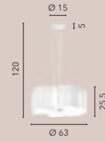
I-IMAGINE-S5 8031440352727 5xE27
