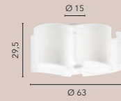
I-IMAGINE-PL5 8031440352734 5xE27
