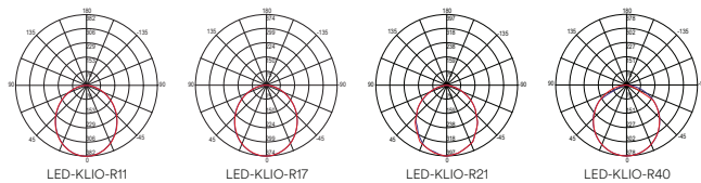
Fotometria del prodotto / Photometric curve
