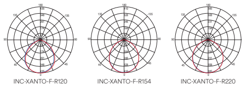
Fotometria del prodotto / Photometric curve
